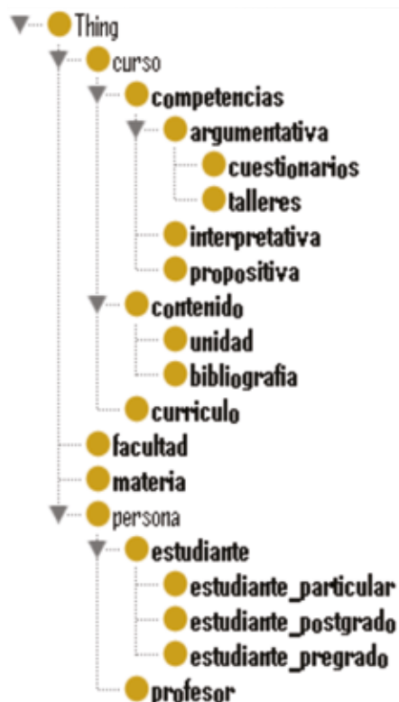
Figura 2. Estructura jerárquica de la ontología. Clases y subclases
